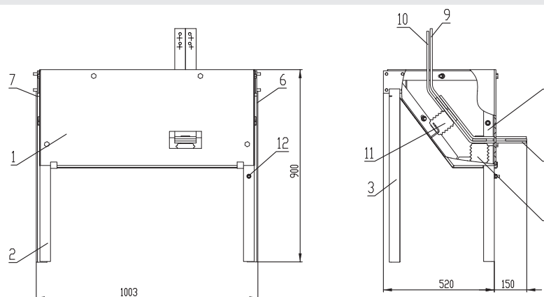
Основание пункта переключений типа ОФ
