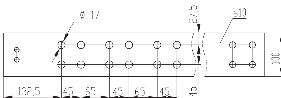
Шина сборная ПП-125 РН-У1
