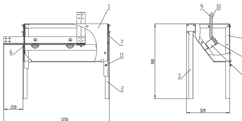
Основание пункта переключений типа ОЛ
