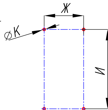
Разметка отверстий для крепления шкафа зажимов Тм
