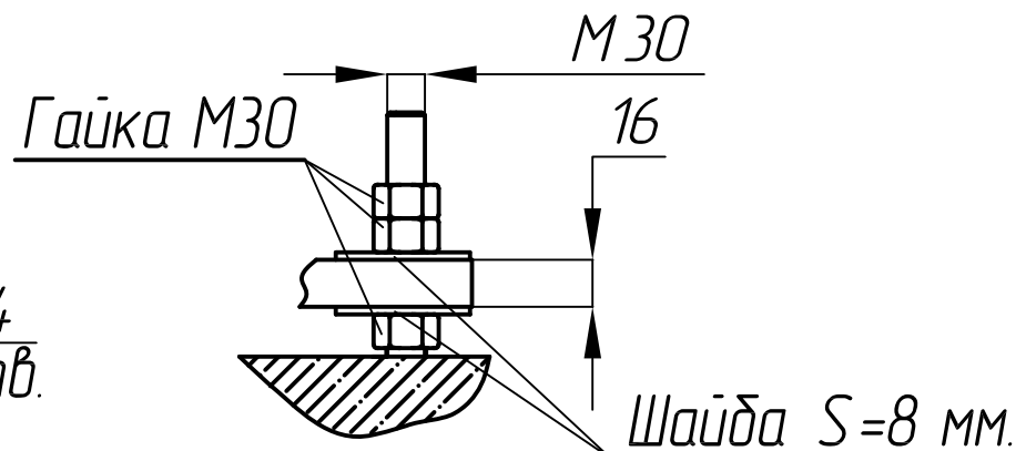
Рисунок 2. Установка блока ТТ-ОП-110 на монолитный фундамент
