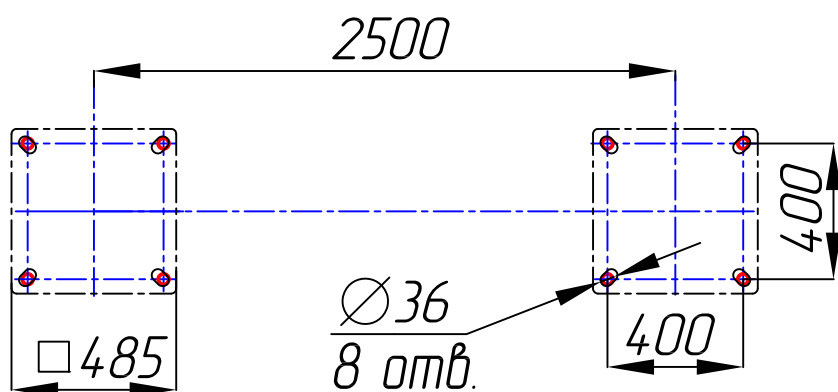
Присоединительные размеры опорных плит стоек к фундаментам
