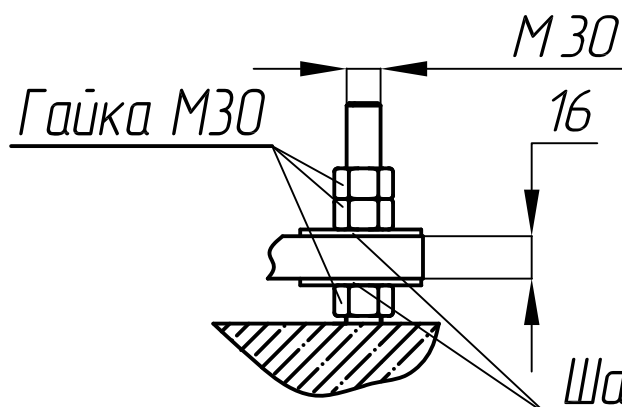
Рисунок 1. Установка блока ТТ-110 на монолитный фундамент
