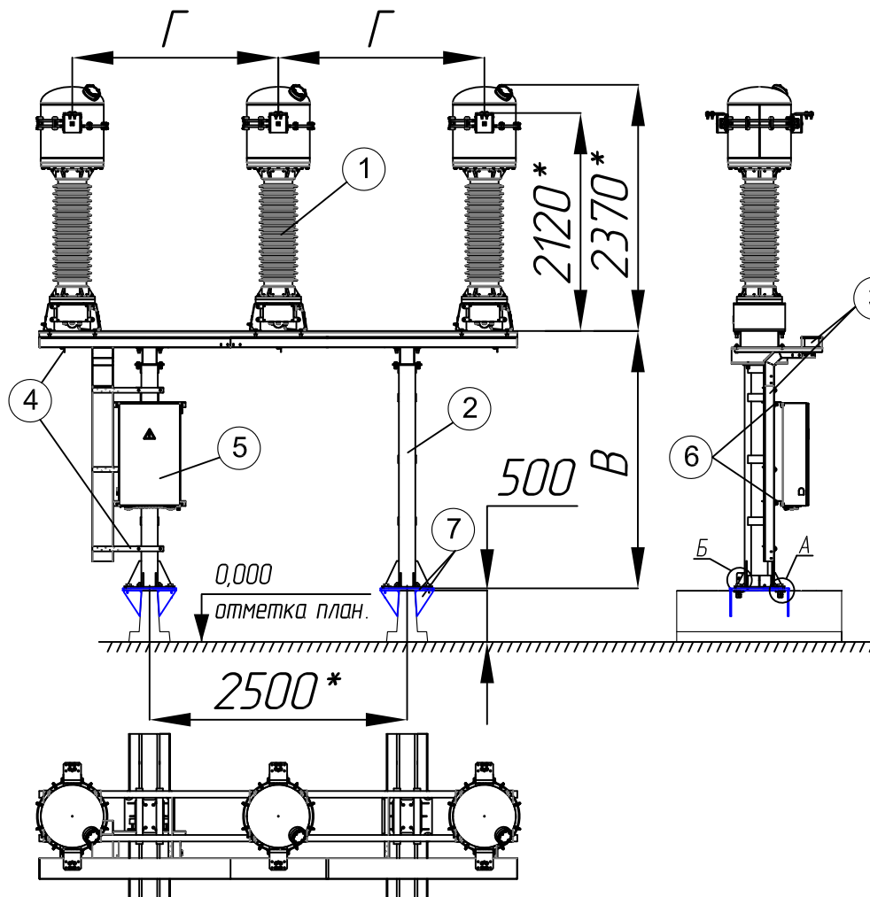
Присоединительные размеры опорных плит стоек к фундаментам
