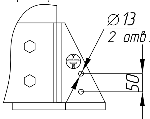
Присоединительные размеры опорных плит стоек к переходной м/к
