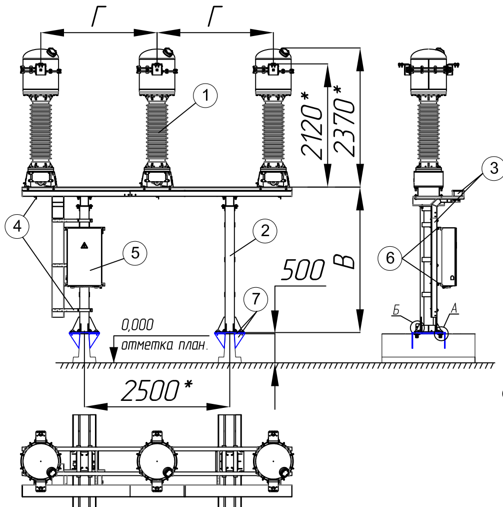
Присоединительные размеры опорных плит стоек к фундаментам
