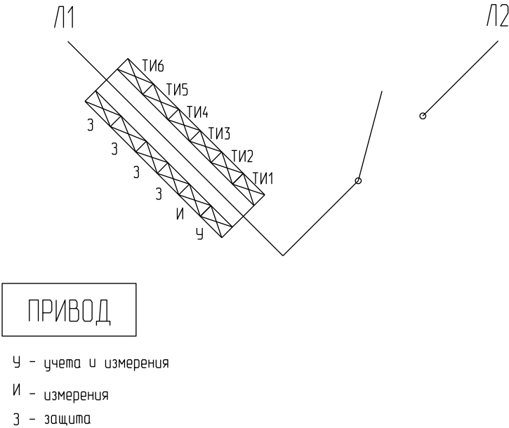
Рисунок 1. Схема расположения максимального количества встроенных трансформаторов тока ТВ в одном полюсе выключателя
